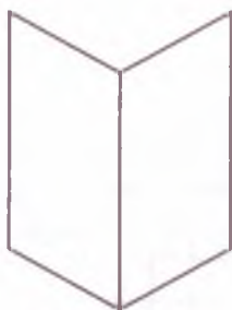
Фигура Маха
